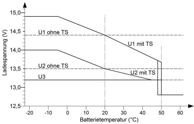
Ladeprogramm Säure „Lead Acid/AGM 1“, IU1oU2oU3
