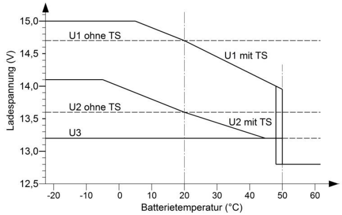
Ladeprogramm „AGM 2“, IU1oU2oU3
