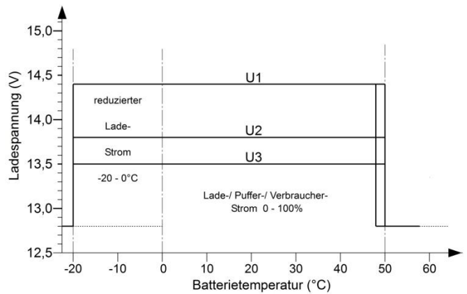
Ladeprogramm „LiFePO4“ 14,4V, IU1oU2oU3
